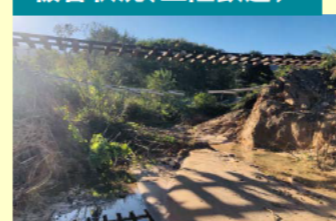
盛土消失（織笠～岩手船越）
